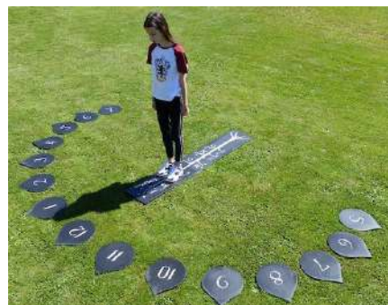
Cadran analemmatique réalisé par Jean-Roch Moreau
